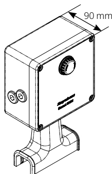
Elexant 3500i elektronischer Thermostat für Rohrmontage
