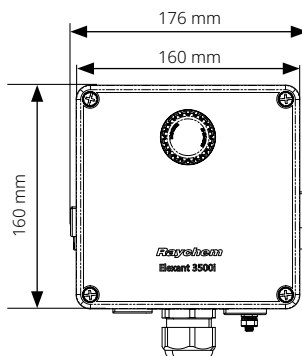
Elexant 3500i elektronischer Wandthermostat
