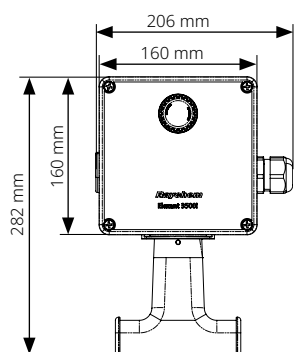
Elexant 3500i elektronischer Thermostat für Rohrmontage
