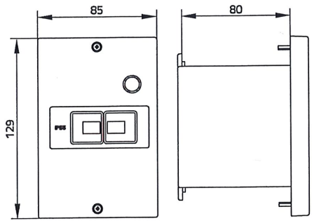
Isolierstoff-Frontplatte MU25-C55
