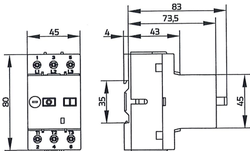
Motorschutzschalter MU25
